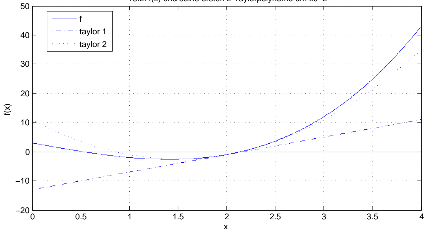
16.2. f(x) und seine ersten 2 Taylorpolynome um x_0=2
